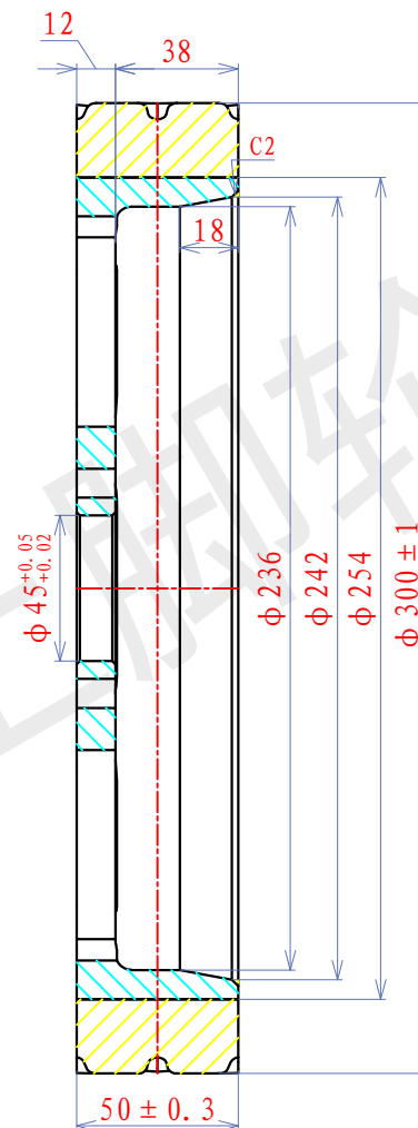
SECTION A-A
